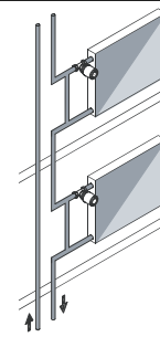
б) однетрубная насосная
