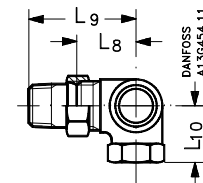
Угловой клапан для монтажа с правой стороны радиатора
