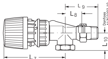
Осевой клапан с термостатическим элементом RA 2991
