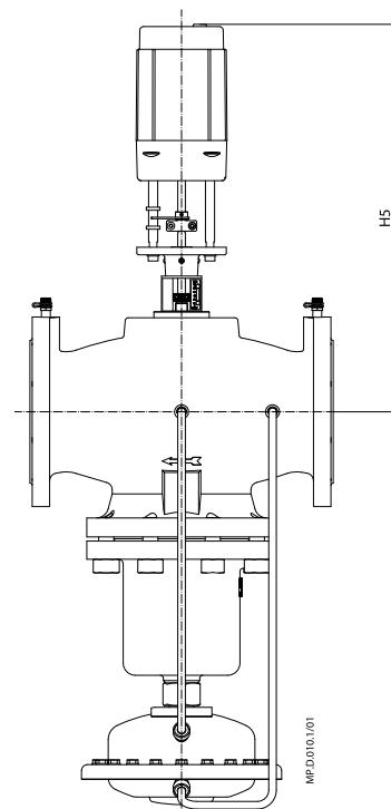
AME 55 QM + AB-QM
